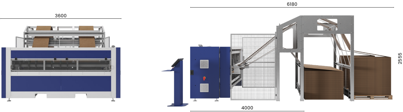
Layoutbeispiel: Smart mit automatischem Einzugssystem
