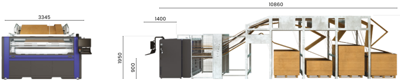
Layoutbeispiel: Nextpro mit automatischem Einzugssystem
